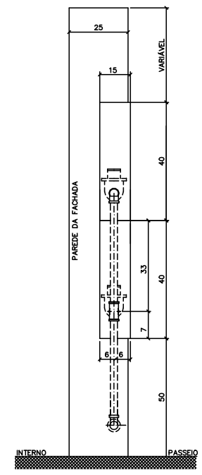
LIGAÇÃO COM CAIXA CORTE A-A
