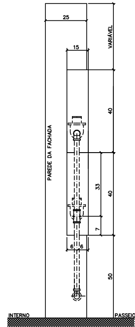
LIGAÇÃO COM CAIXA CORTE A-A
