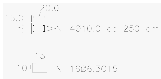
Figura 2a: Armadura dopilar de concreto.
