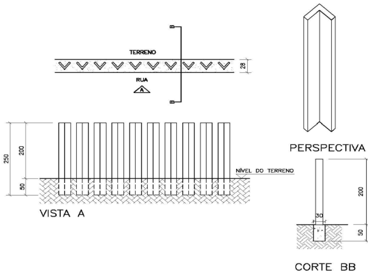
Figura 1: Demonstração esquemática do muro pré-moldado com calhas de concreto em "V".
