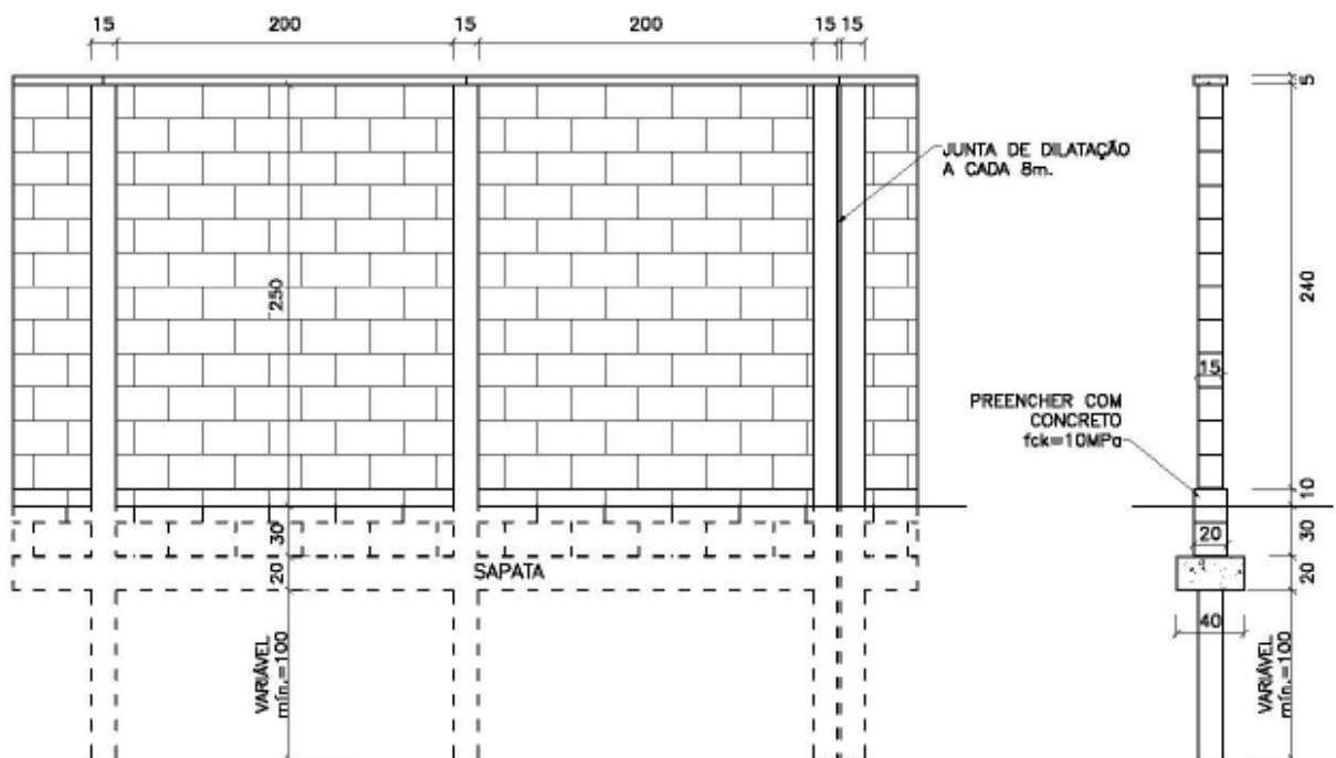
Figura 2: Demonstração esquemática do muro em bloco de concreto aparente.
