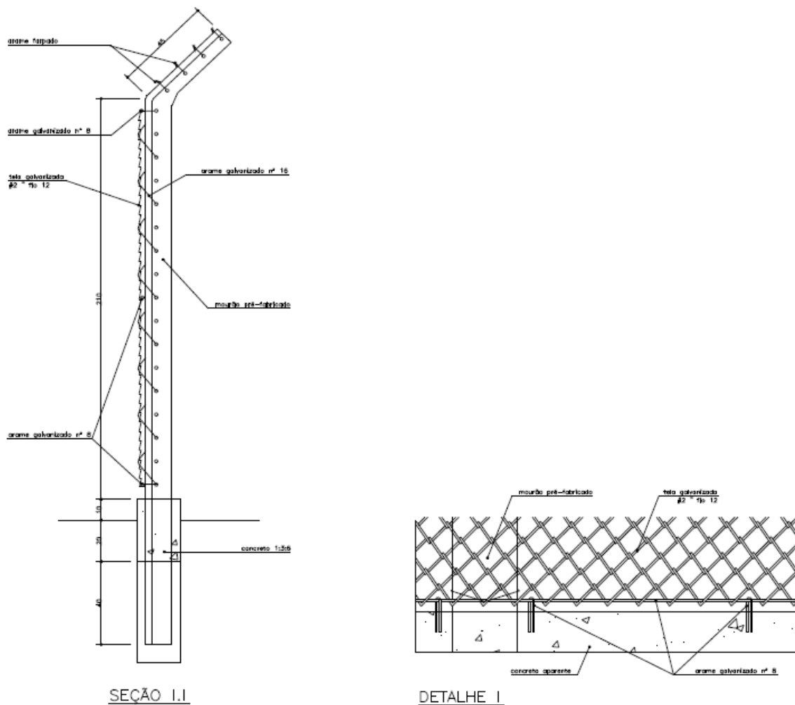
Figura 4: Demonstração esquemática da cerca com tela galvanizada.
