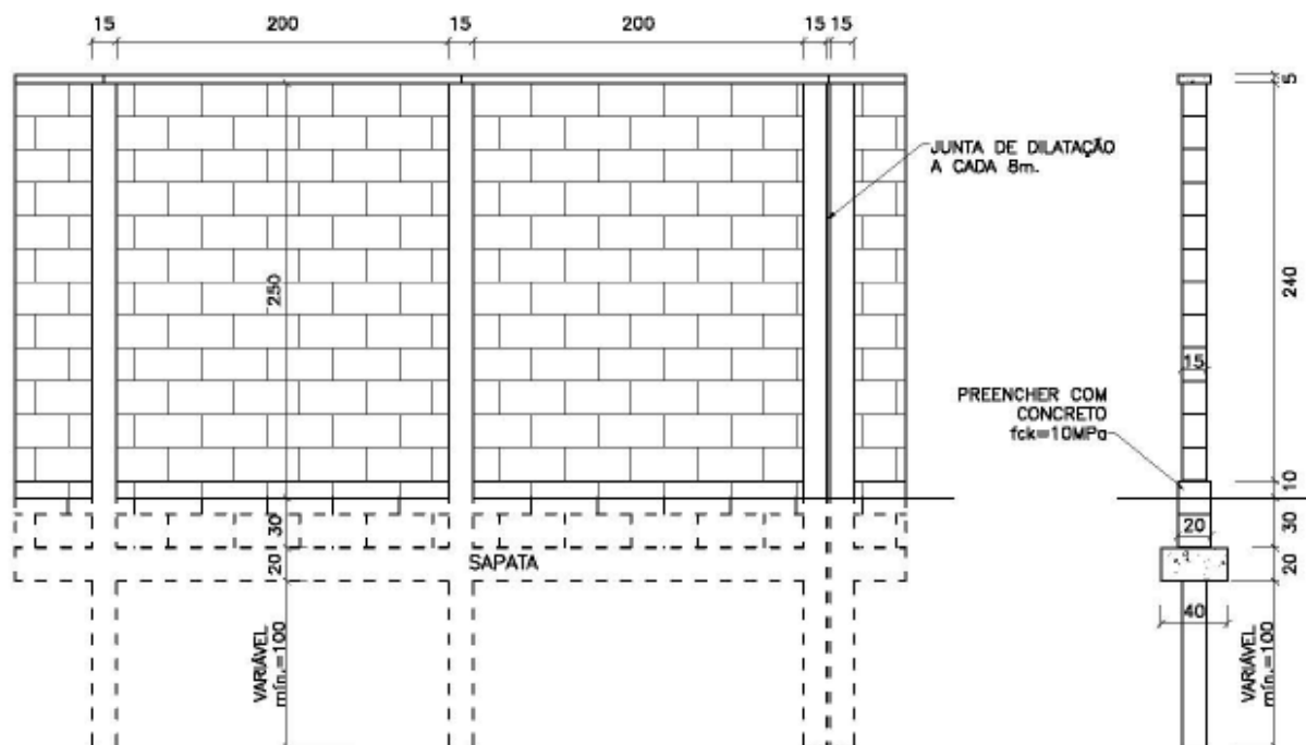
Figura 2a: Demonstraç o esquem tica do muro em bloco de concreto aparente.
