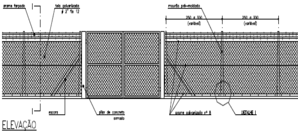
Figura 4: Elevação esquemática da cerca com tela galvanizada.
