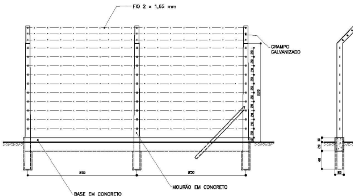
Figura 2: Demonstração esquemática da cerca com arame farpado.
