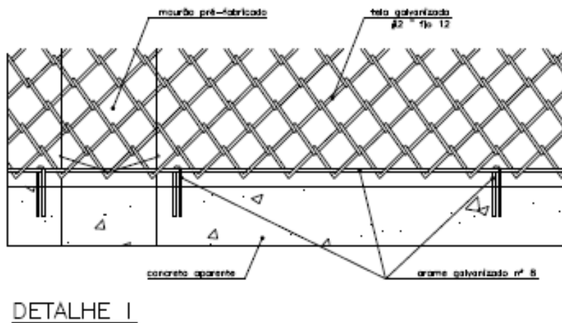
3a: Detalhe esquemático da da tela galvanizada inferior.
